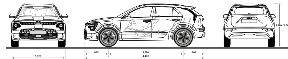
Masse EV (mm)
